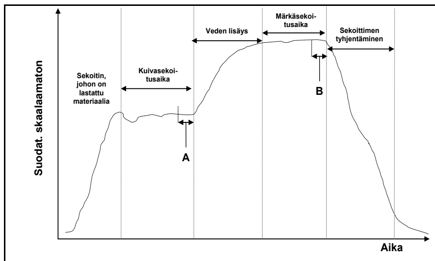
Kuva 5: Tyypillinen kosteuskäyrä
