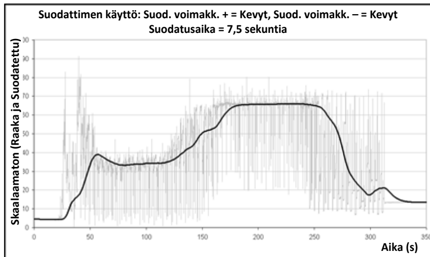
Kuva 8: Raakasignaalin suodatus (2)
