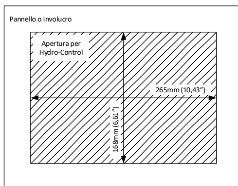
Figura 6: Apertura sul pannello per il dispositivo Hydro-Control
