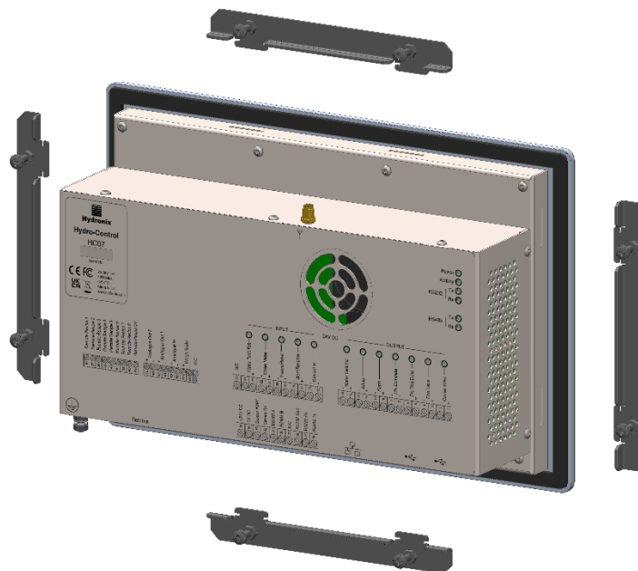
Figura 5: Staffe di montaggio
