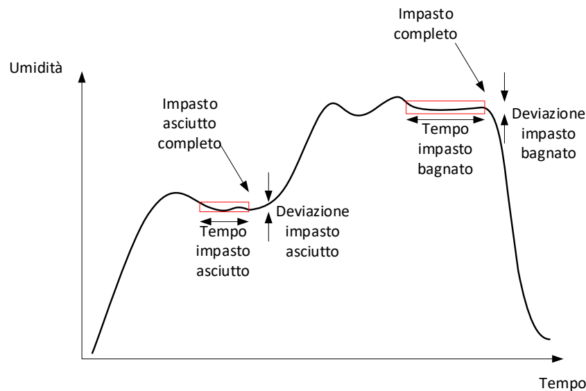
Figura 74: Traccia dell'impasto da cui risultano le impostazioni Auto-Track
