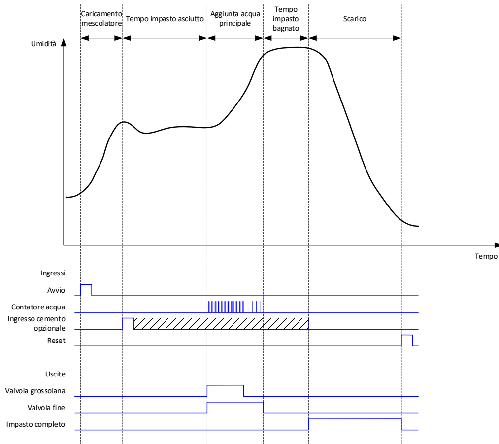
Figura 71: Ciclo d'impasto con lo stato degli ingressi/delle uscite
