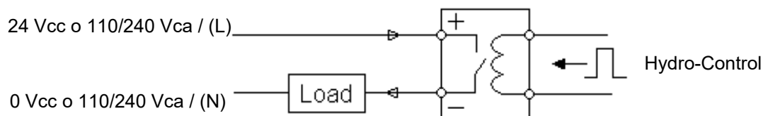
Figura 12: Schema di cablaggio delle uscite digitali
