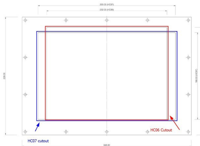
Figura 7: Allineamento delle aperture sul pannello per le versioni HC06 e HC07
