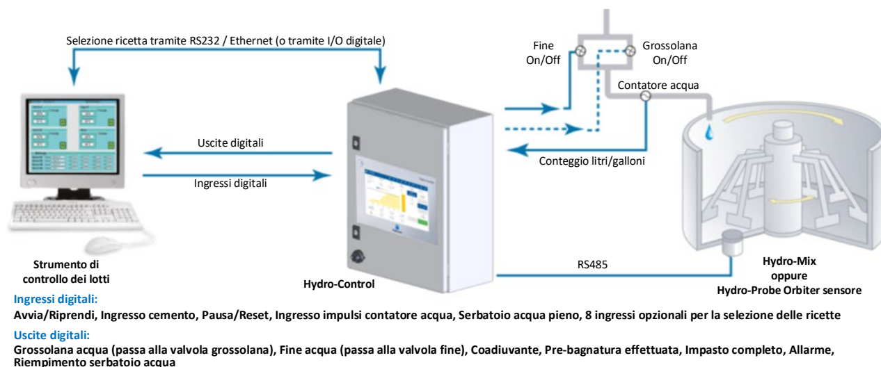
Figura 2: Esempio di implementazione di Hydro-Control
