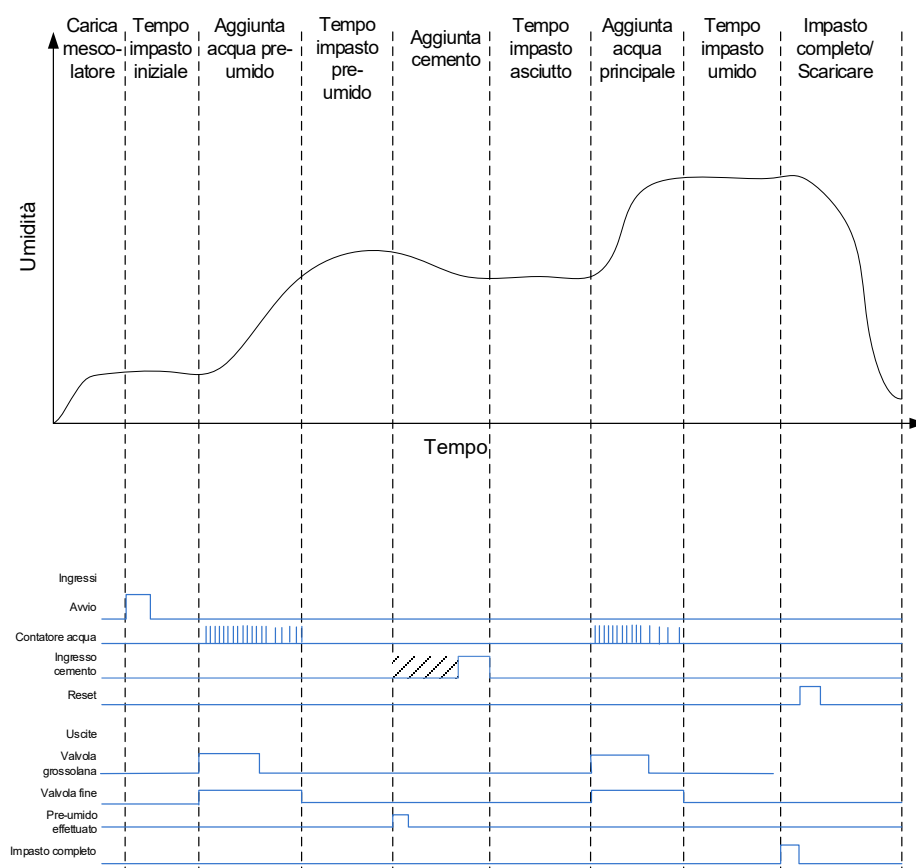
Figura 70: Ciclo d'impasto completo
