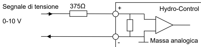
Figura 20: Connessione di segnale di tensione a Ingresso analogico
