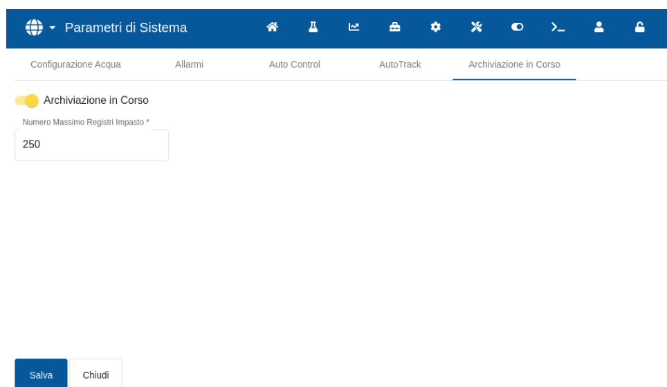
Figura 37: Pagina Archiviazione
