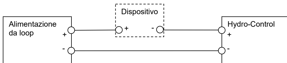
Figura 18: Collegamento di dispositivo alimentato da loop
