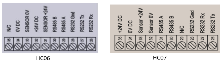
Figura 9: Differenze di piedinatura del connettore a 10 pin della versione HC06 rispetto alla HC07
