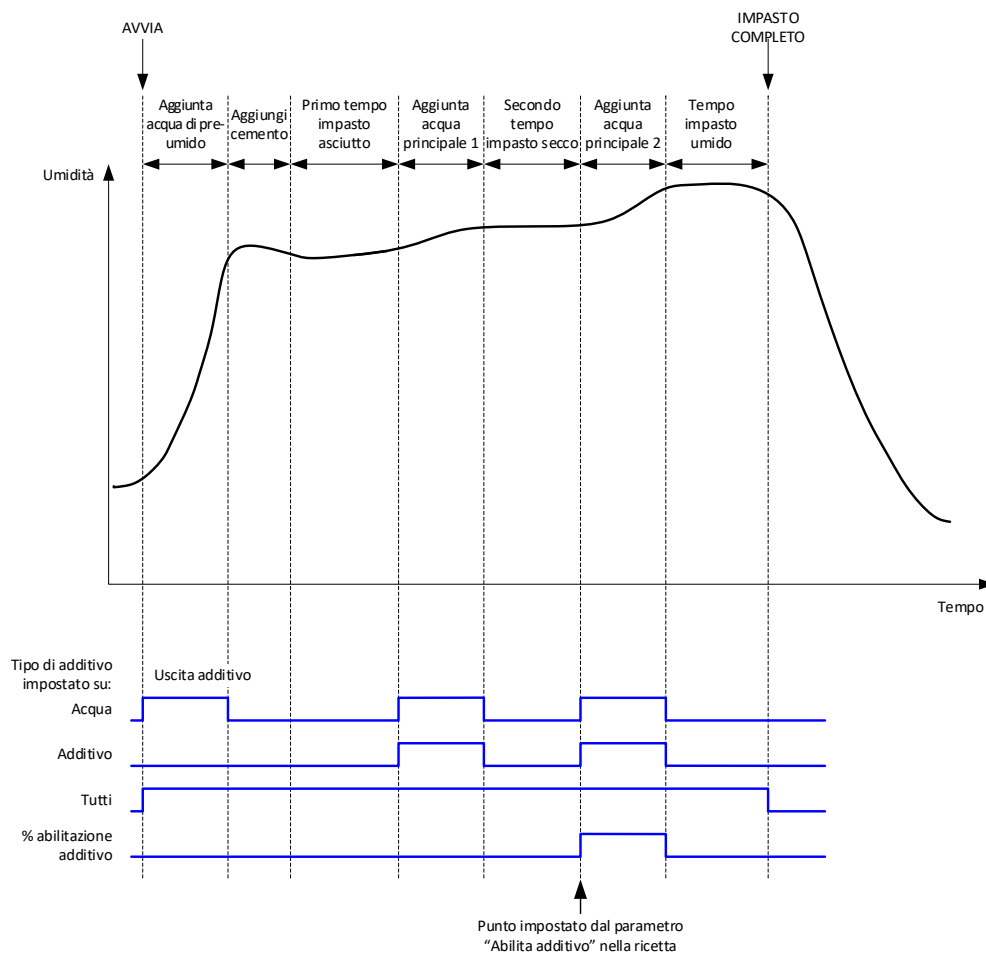
Figura 73: Segnale di uscita additivo durante un ciclo d'impasto in 2 fasi
