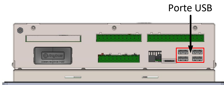
Figura 77: Posizione delle porte USB
