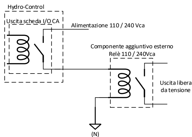
Figura 16: Attivazione di un dispositivo CC utilizzando un'uscita di scheda I/O CA
