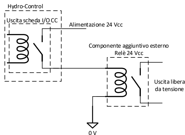
Figura 15: Attivazione di un dispositivo CA utilizzando un'uscita di scheda I/O CC
