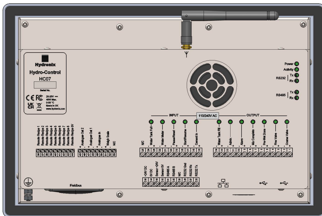
Figura 4: Retro del dispositivo Hydro-Control
