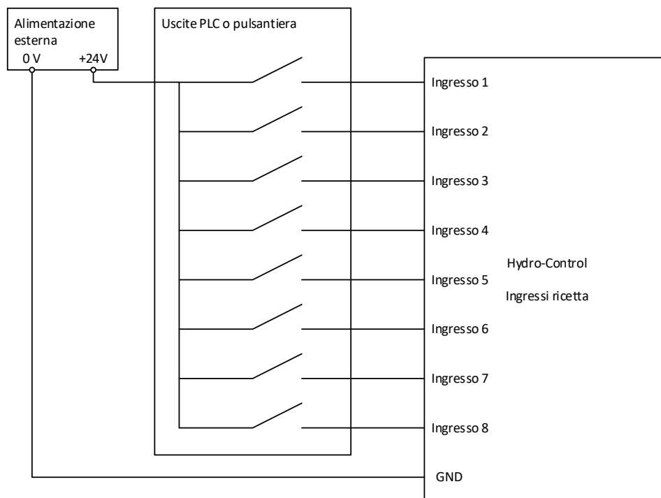
Figura 22: Cablaggio di ingressi di selezione delle ricette
