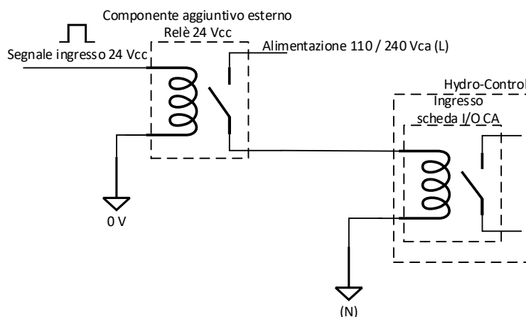
Figura 13: Collegamento di un segnale di ingresso CC a una scheda di ingresso CA
