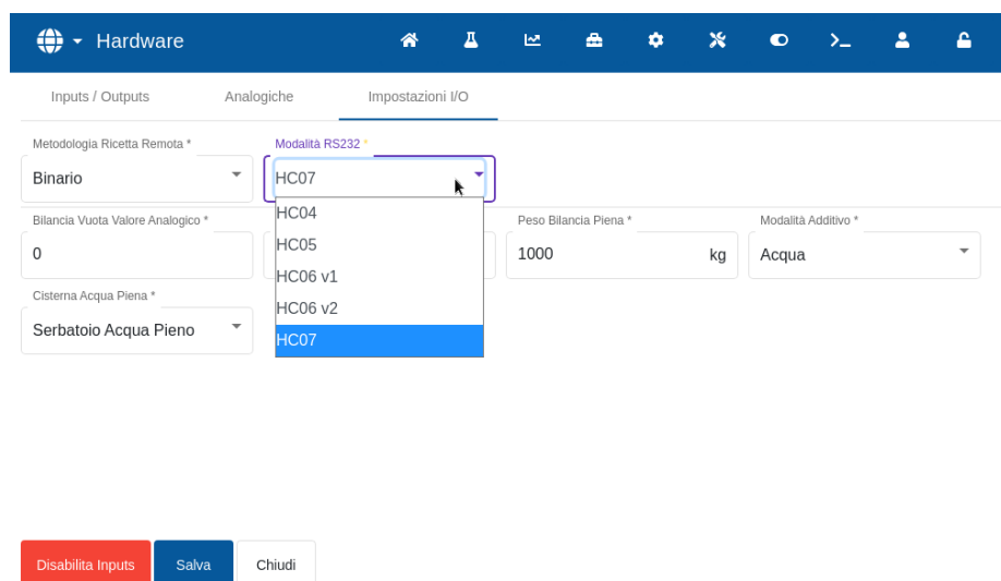
Figura 76: Opzioni di comunicazione RS232
