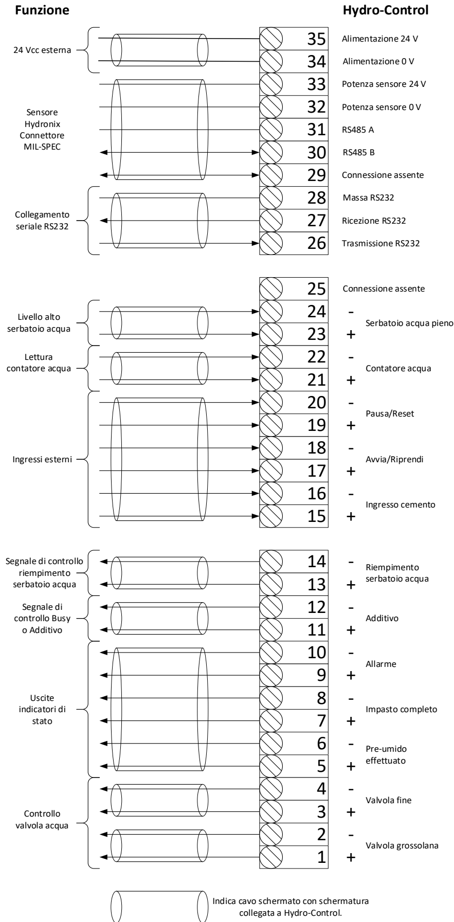
Figura 69: Interconnessioni di sistema
