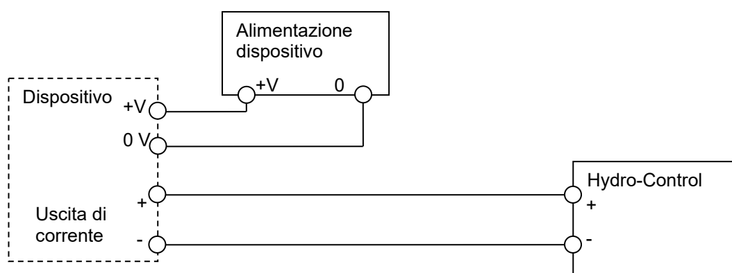
Figura 19: Collegamento del loop di corrente di un dispositivo alimentato esternamente
