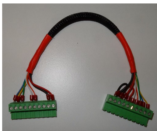
Figura 10: Cavetto adattatore per cablaggio dalla versione HC06 alla HC07
