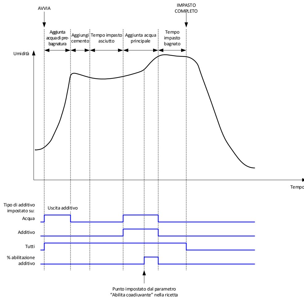
Figura 72: Segnale di uscita additivo durante un ciclo d'impasto normale
