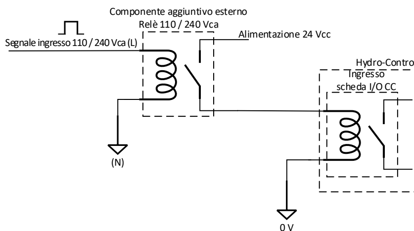
Figura 14: Collegamento di un segnale di ingresso CA a una scheda di ingresso CC
