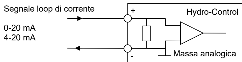
Figura 17: Schema di cablaggio del loop di corrente di ingresso analogico
