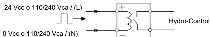
Figura 11: Schema di cablaggio degli ingressi digitali
