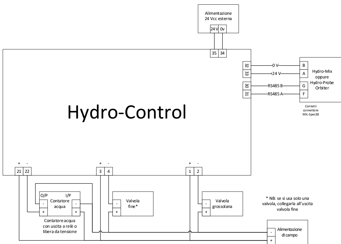
Figura 67: Esempio di schema di cablaggio per il funzionamento manuale dell'impianto
