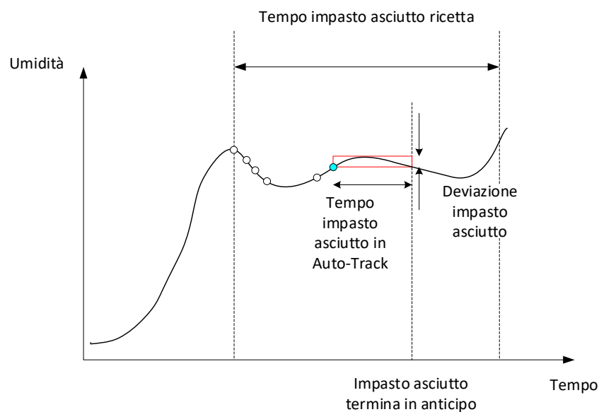
Figura 75: Esempio di parametro Auto-Track per la fase d'Impasto asciutto
