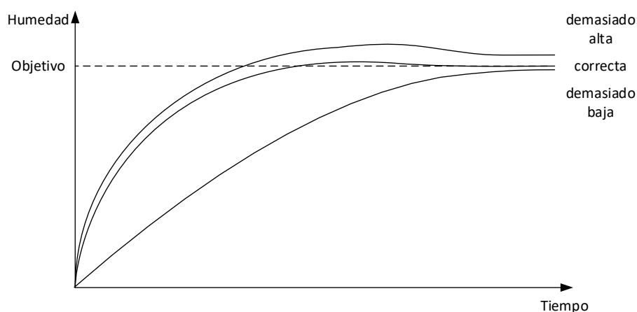
Figura 58: El efecto de cambiar la ganancia derivada
