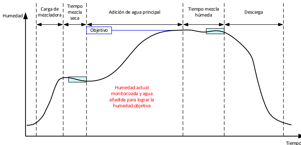
Figura 55: Humedad durante el modo Automático
