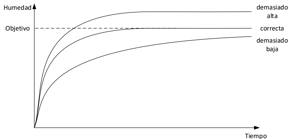
Figura 56: El efecto de cambiar la ganancia proporcional
