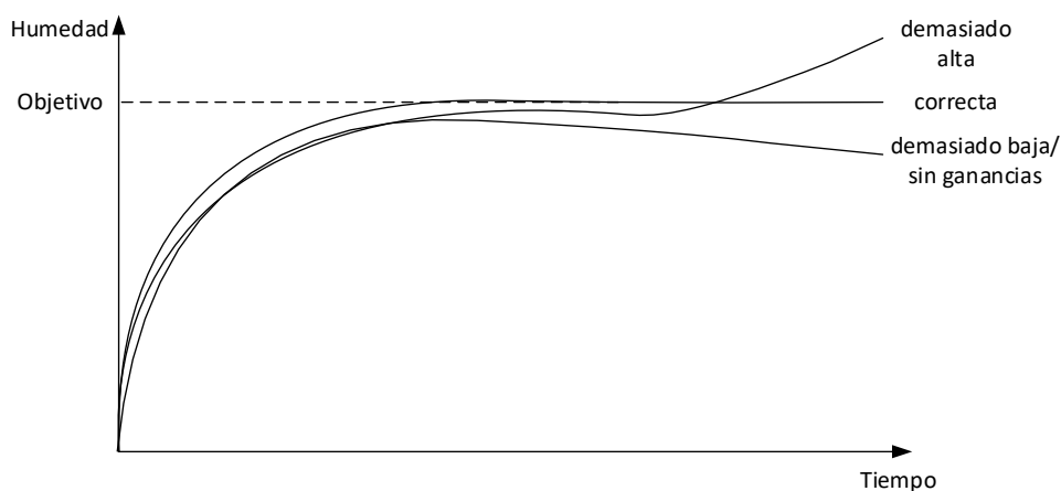
Figura 57: El efecto de cambiar la ganancia integrada
