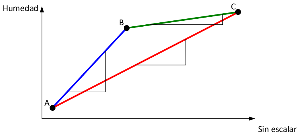
Figura 60: Las líneas de calibración del ciclo del modo Preestablecido en dos pasos
