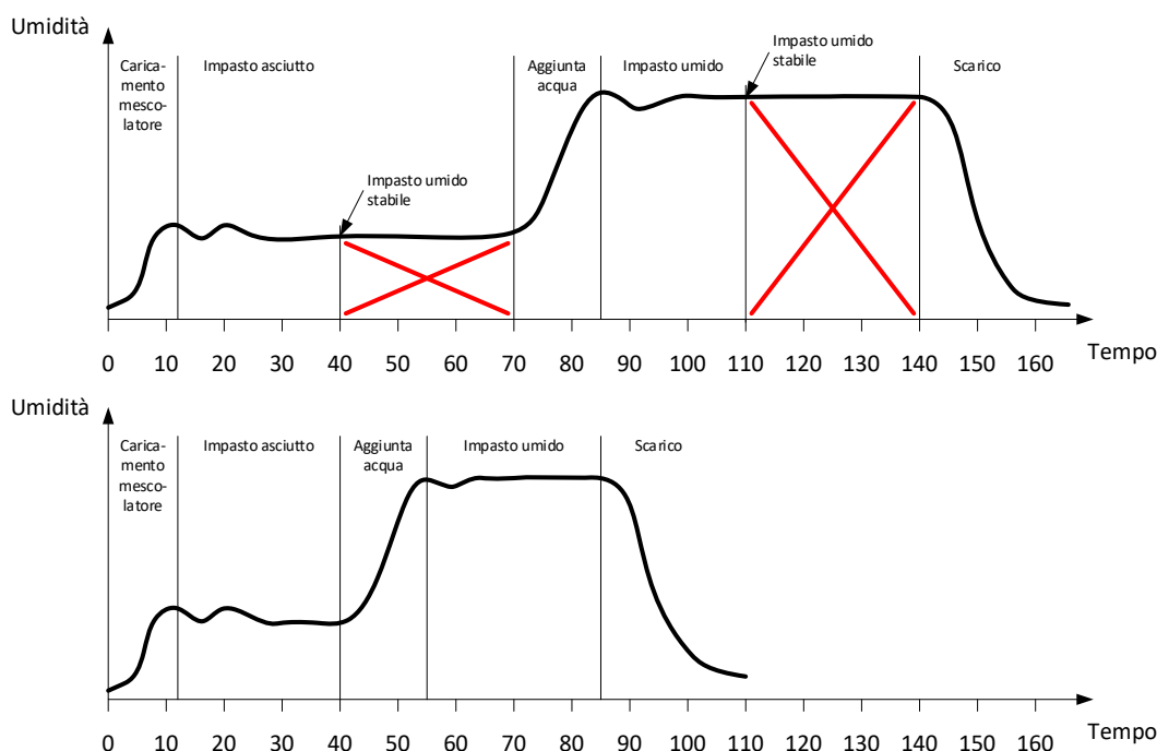
Figura 44: Prolungamento dei tempi di impasto per la calibrazione
