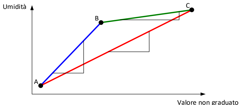
Figura 60: Linee di calibrazione ricavate dal ciclo in Modalità Preset in 2 fasi
