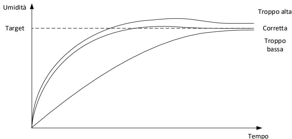
Figura 58: Effetto della variazione del Guadagno derivativo
