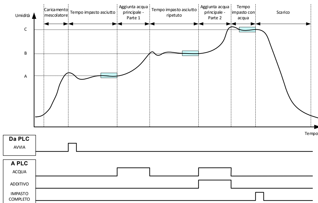
Figura 59: Ciclo in Modalità Preset in 2 fasi
