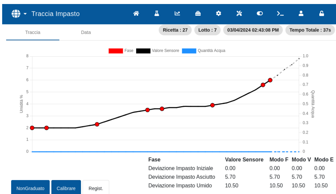
Figura 41: Schermata Tracciato impasto per un sensore precedente
