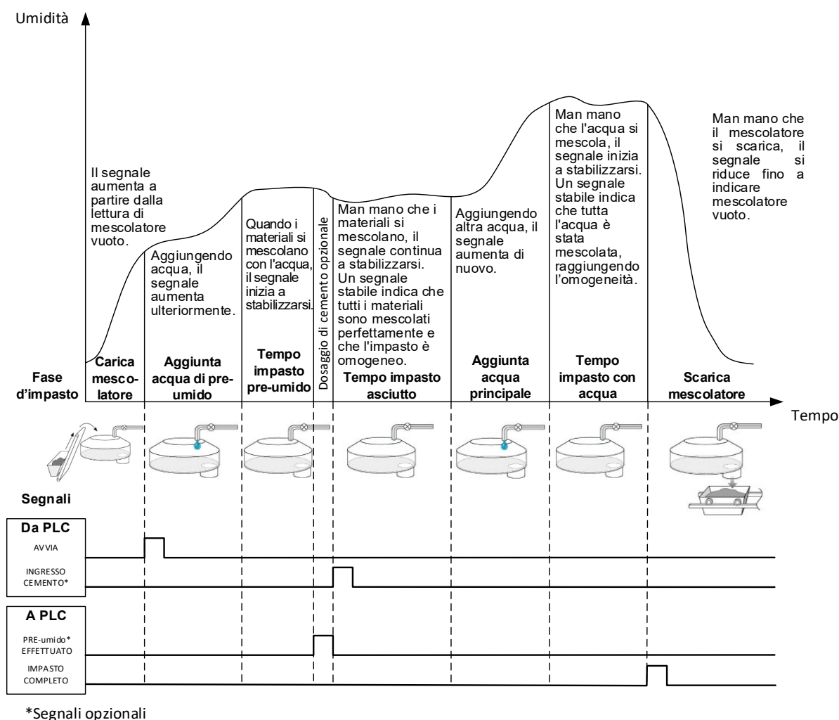
Figura 26: Ciclo d'impasto con fase di pre-umido
