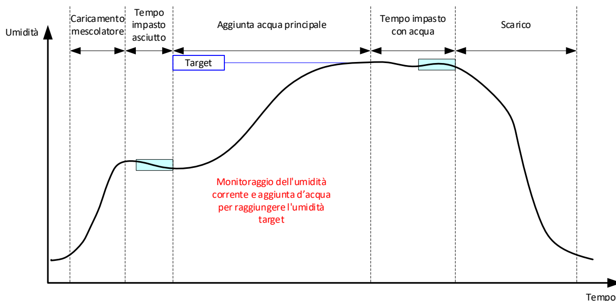
Figura 55: Umidità durante la Modalità CALC
