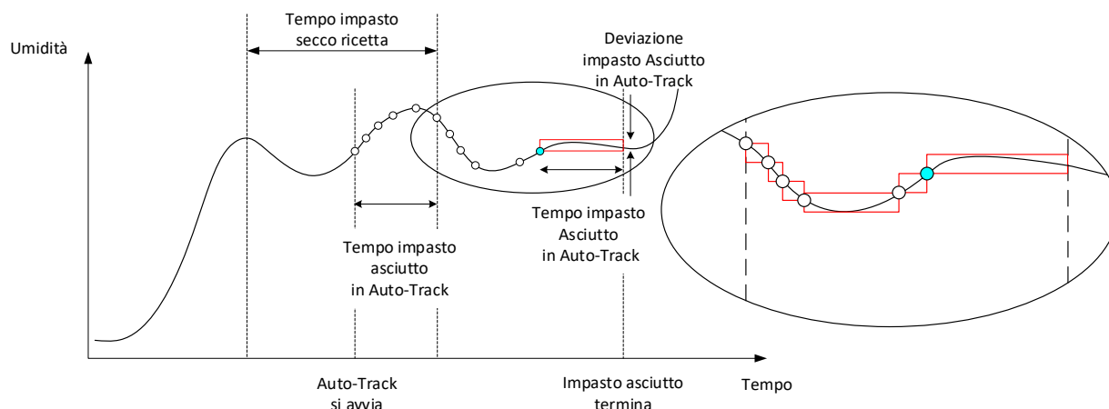
Figura 61: Tracciato impasto che mostra la funzione Auto-Track
