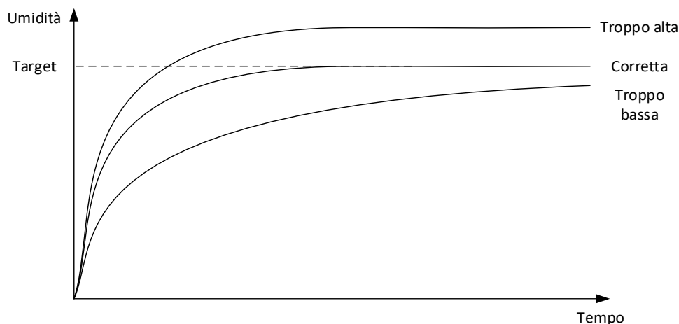
Figura 56: Effetto della variazione del Guadagno proporzionale
