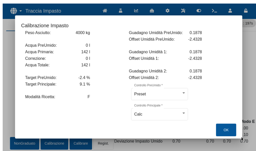
Figura 51: Riepilogo dei parametri di calibrazione
