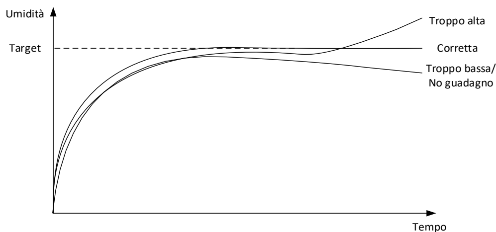
Figura 57: Effetto della variazione del Guadagno integrale
