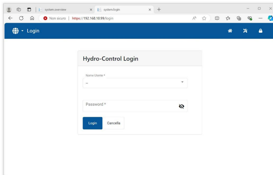
Figura 73: Schermata Login
