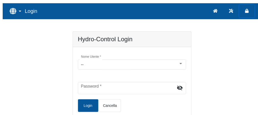
Figura 18: Schermata Login
