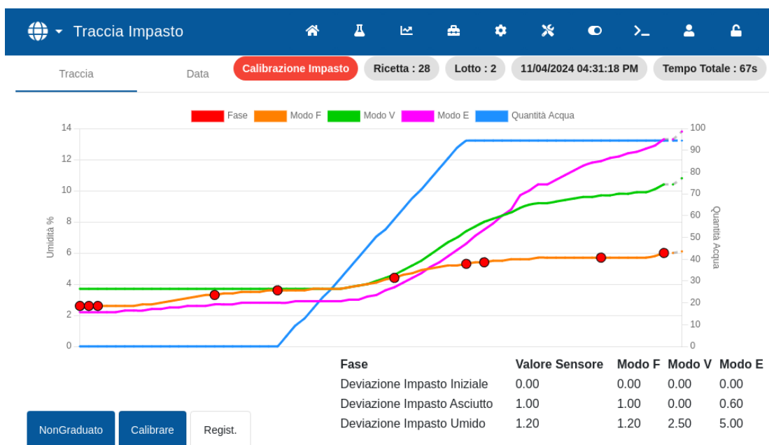
Figura 40: Schermata Tracciato impasto
