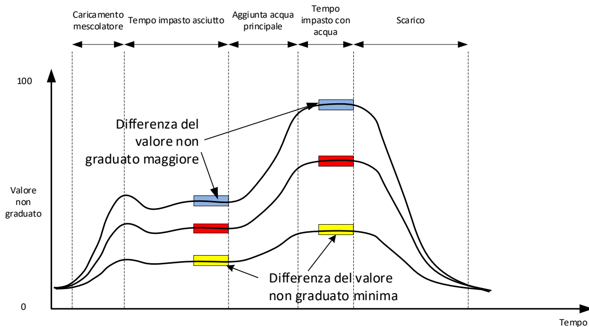
Figura 54: Confronto tra modi di misurazione
