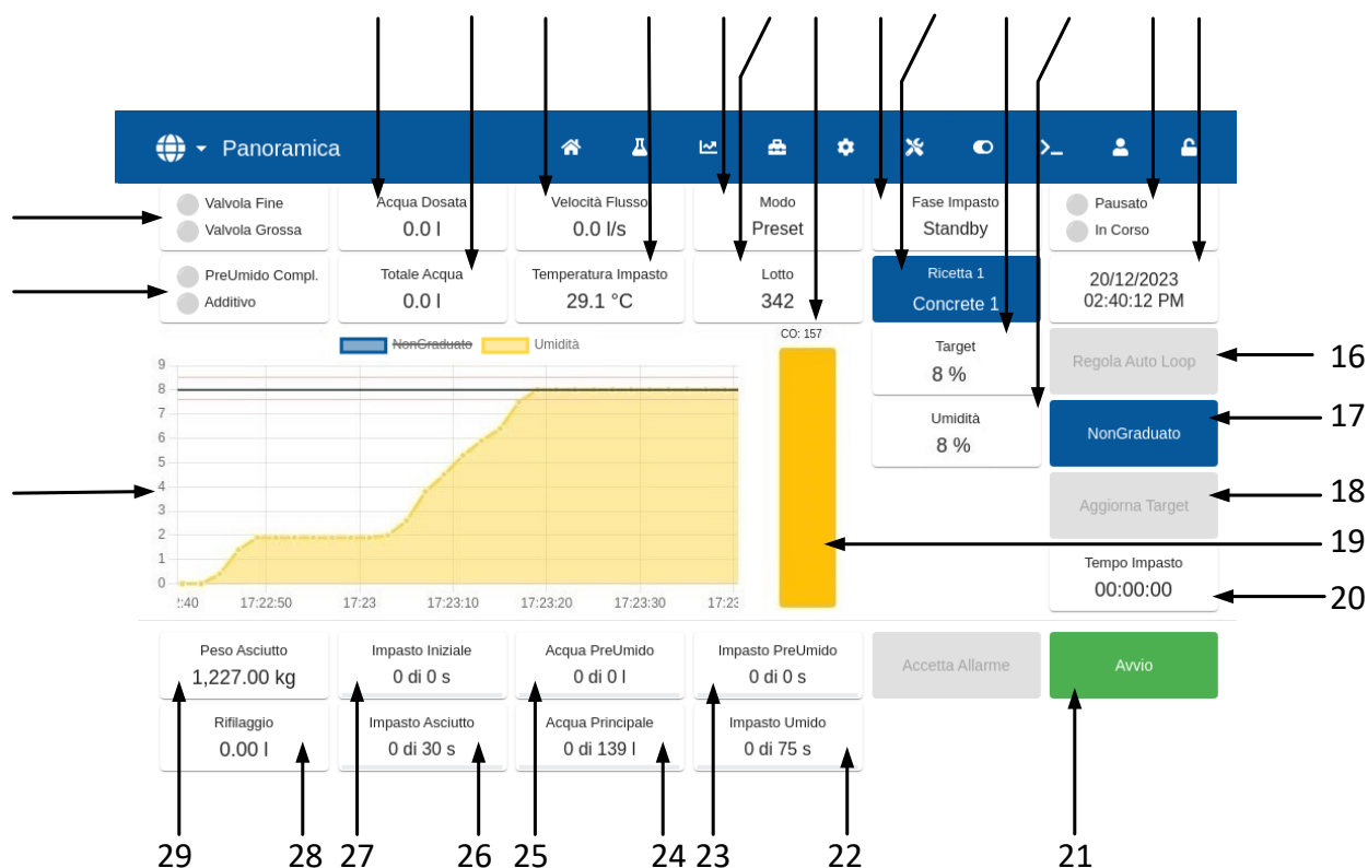
Figura 6: Schermata Panoramica di Hydro-Control
